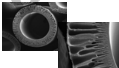
MEDISULFONE®: sezione e morfologia di una singola fibra capillare cava
